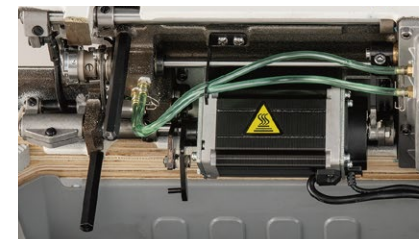
自动切线&自动抬压脚脉冲马达
